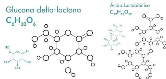
Figura 10. Estructuras moleculares de los Polihidroxiácidos
