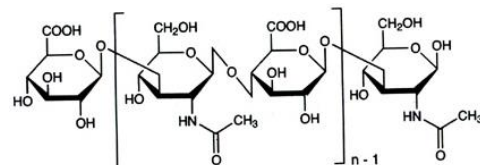
Figura 9. Estructura química básica del Ácido hialurónico.
